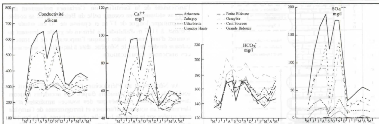
Figure 4 : Evolution de la conductivité, des ions Ca^{2+} , HCO_3^- et SO_4^{2-} de huit grandes émergences des Arbailles (Année 95-96).
