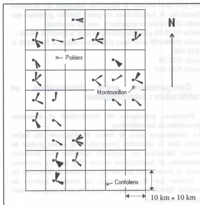
figure 4 : Répartition spatiale des directions préférentielles de karstification à l'échelle du département de la Vienne (programme DENS, DELAY et al., 1993).
