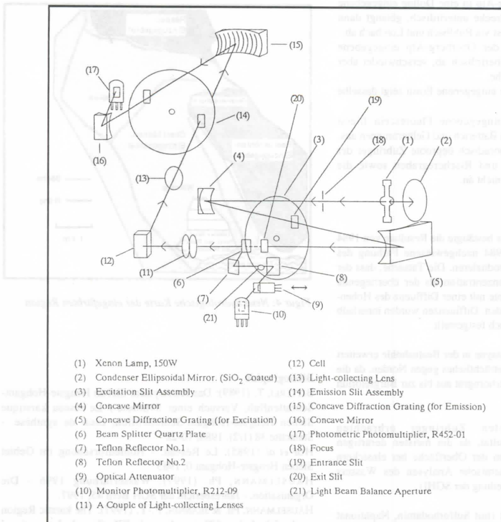
Figur 3: Shimadzu RF5001-PC. Die Funktionsweise und der Aufbau entspricht annähernd dem des LS-2B.
