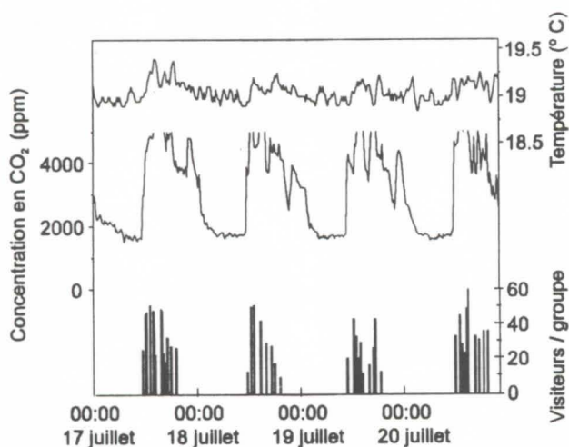
Figure 4.- Concentration en CO 2 de l'air, température de l'air et nombre de visiteurs par groupe dans la Verrerie de Dieu.
