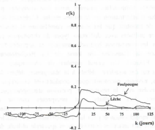
Figure 3 : Corrélogrammes croisés des chroniques de débits
