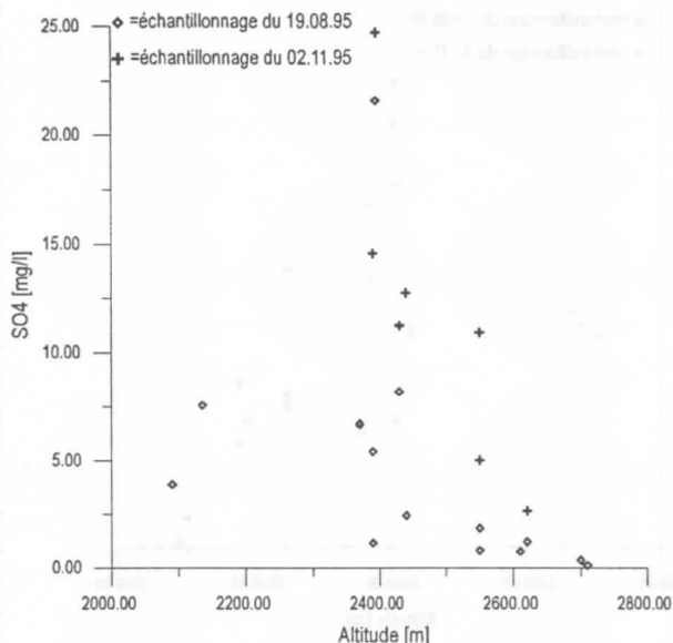
Figure 3: Evolution de la concentration en éléments majeurs (Ca, Mg, SO 4 ) en fonction de l'altitude et des conditions hydrodynamiques.
