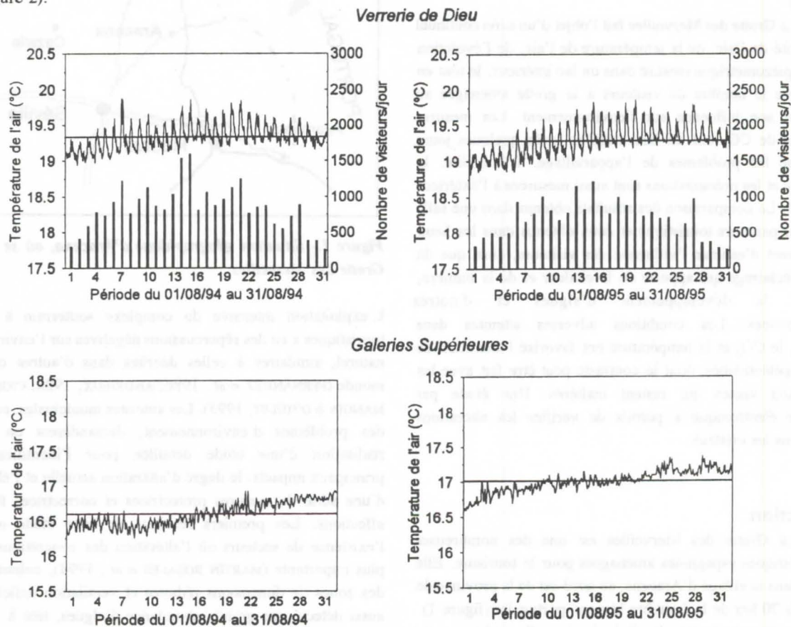
Figura 3.- Enregistrements continus de température de l'air et entrée de visiteurs dans la Verrerie de Dieu et les Galeries Supérieures, correspondant au mois d'août 1994 et août 1995.
