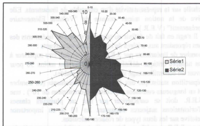
figure 3 : Répartition statistique des directions préférentielles de karstification à l'échelle du département de la Vienne (Série 1 : pourcentages en longueurs cumulées de linéaments ; Série 2 : pourcentages en nombre de linéaments).
