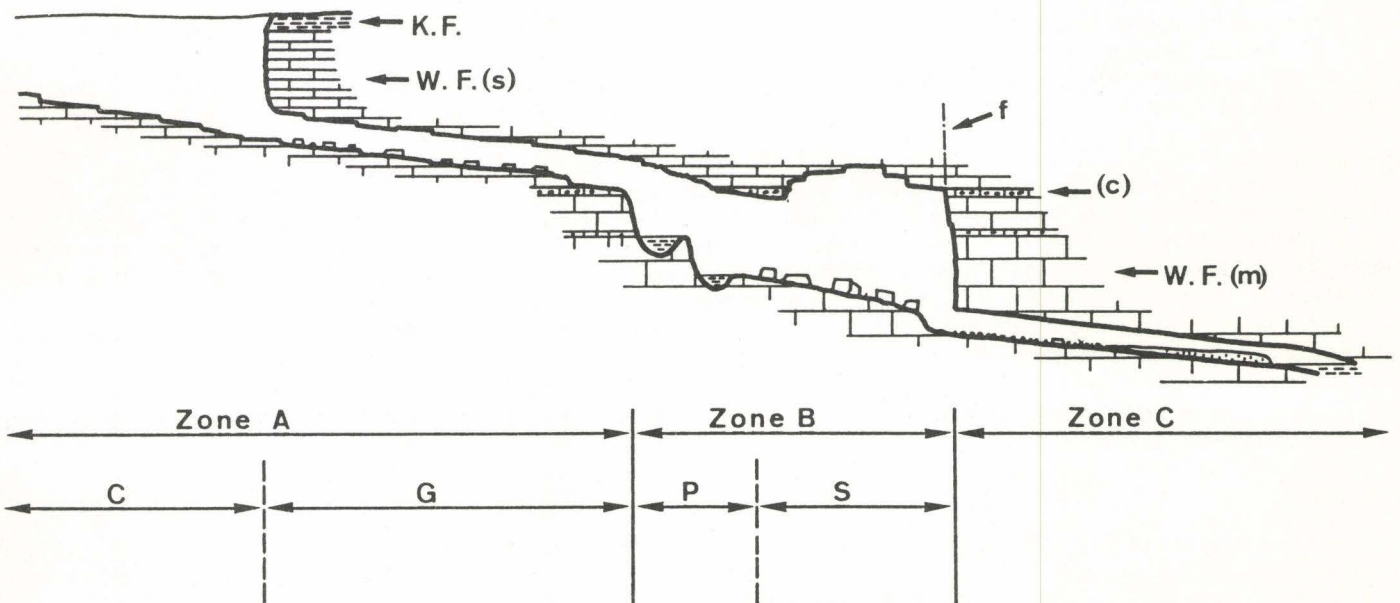
Figure 6. Coupe synthétique type d'un gouffre-grotte.
