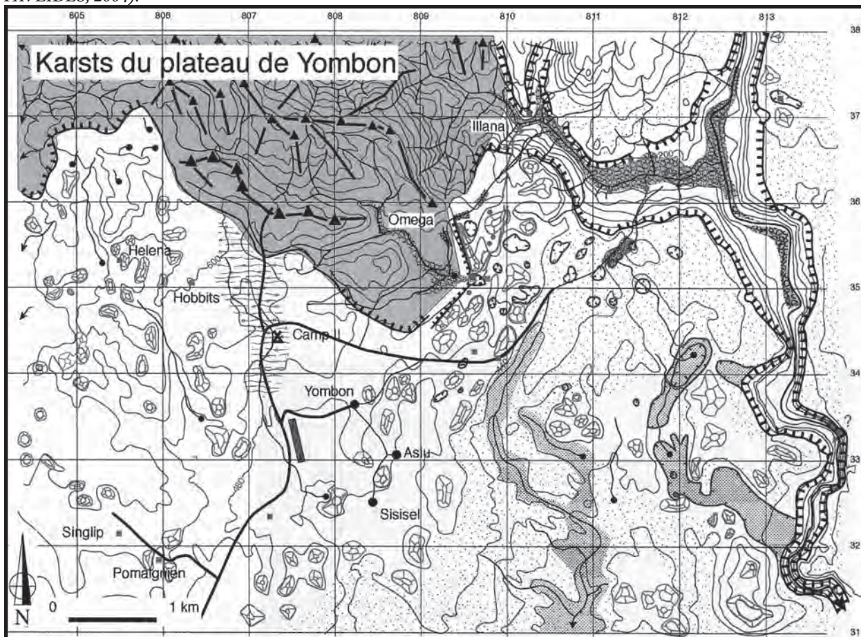
Figure 2: Aperçu géomorphologique des karsts du plateau de Yombon et situation des cavités explorées (d'après Collectif Niugini 2001).
