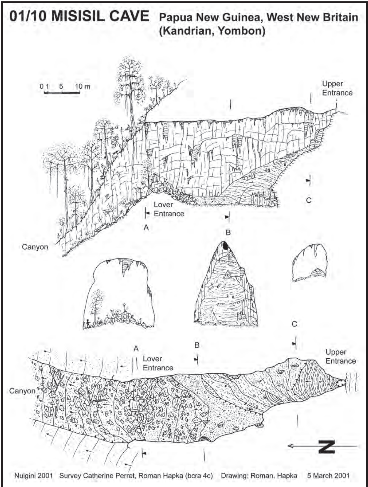
Figure 4: Topographie de la grotte de Misisil.
